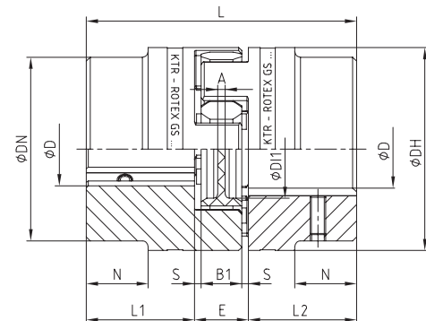
ROTEX® GS 42 - 90
