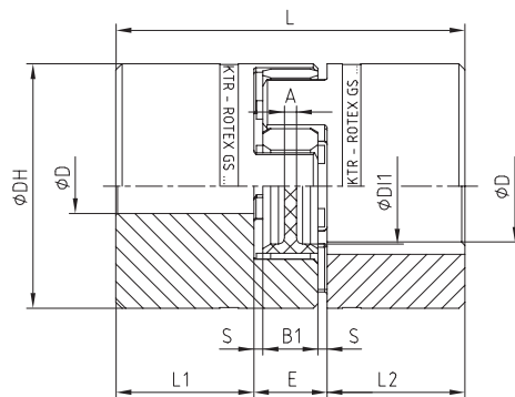
ROTEX® GS 5 - 38
